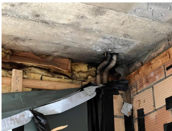
Dalle hybride entre le rez et l'étage, pour partie en béton, pour partie en poutraison
